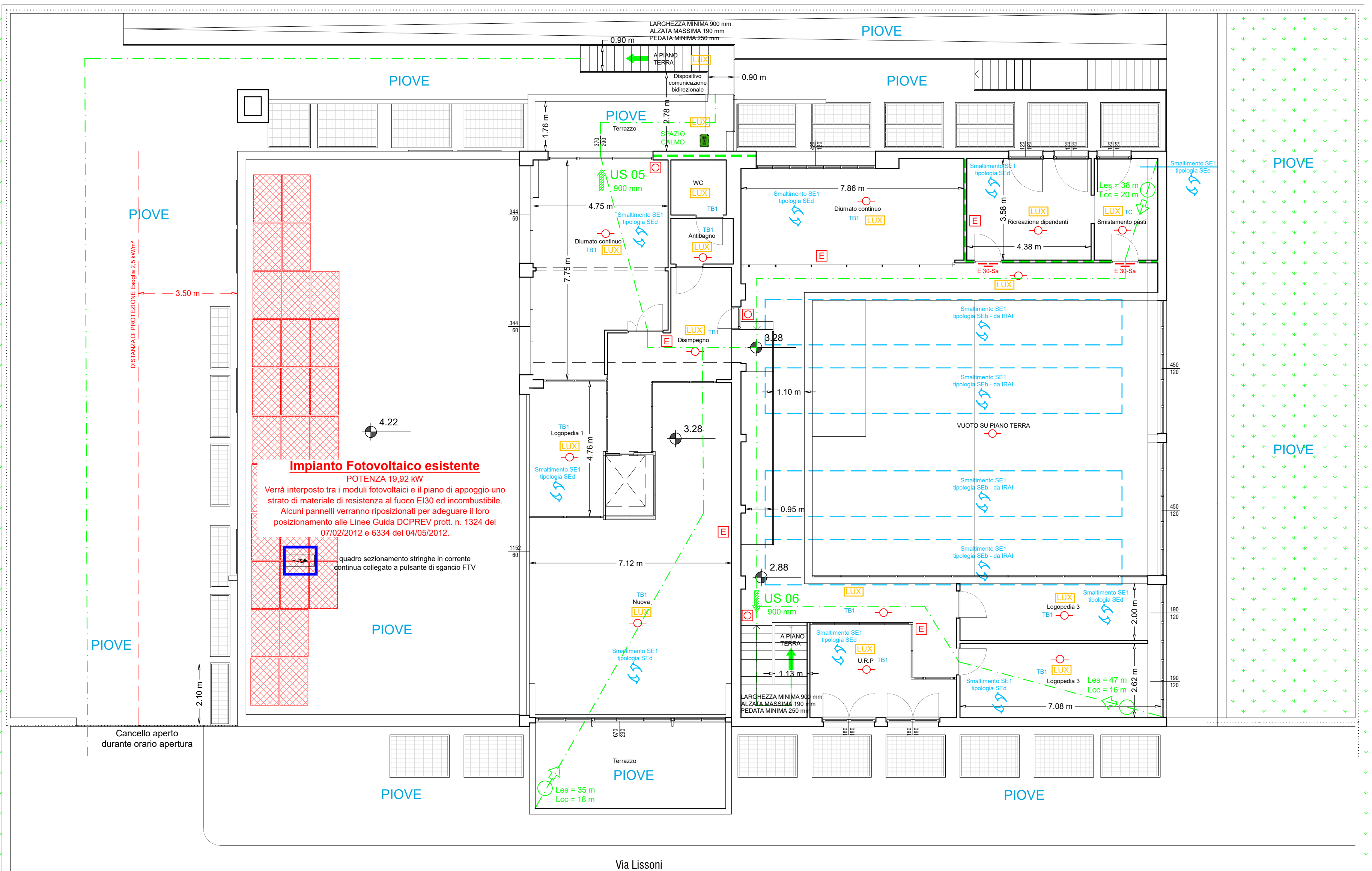
PIANO PRIMO
